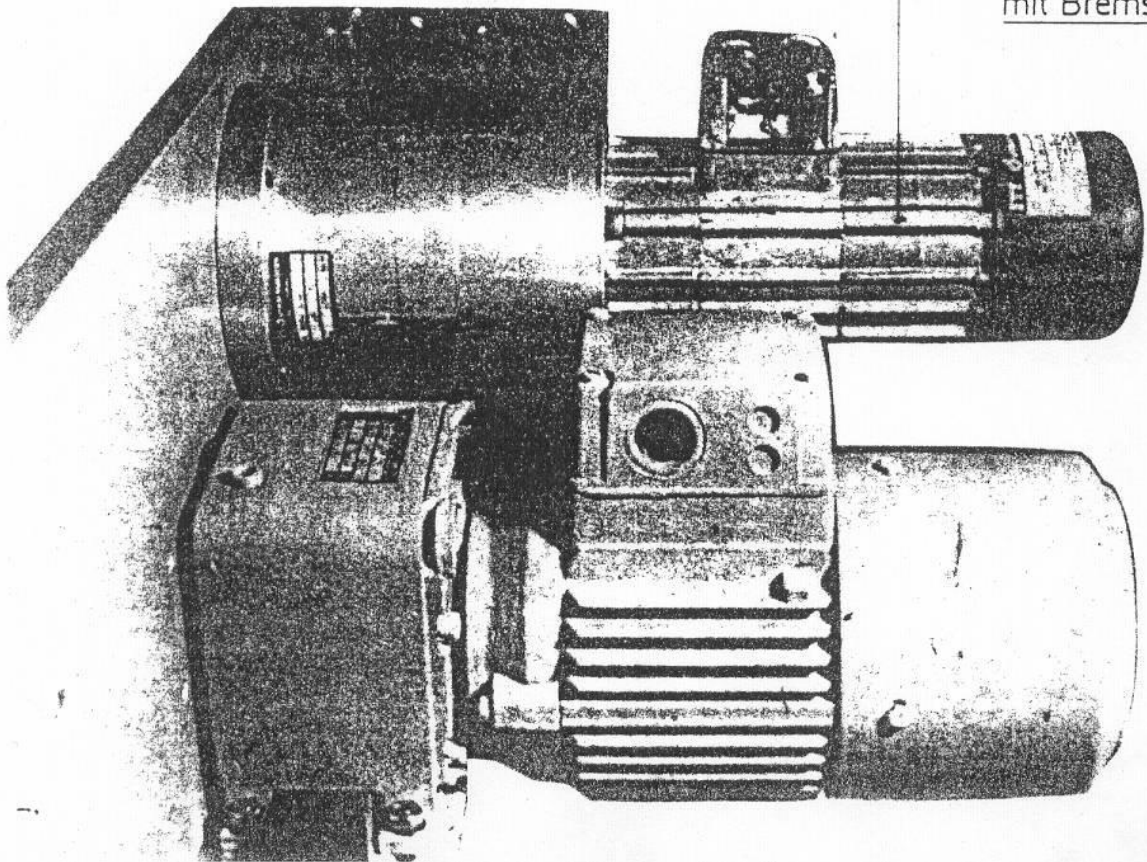
11 036 Drehstrommotor mit Bremse
